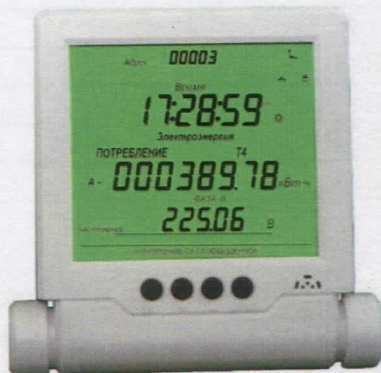
Рисунок 9 - Общий вид дистанционного индикаторного устройства
