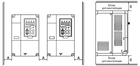
Рис. 4-1 Монтажная схема
